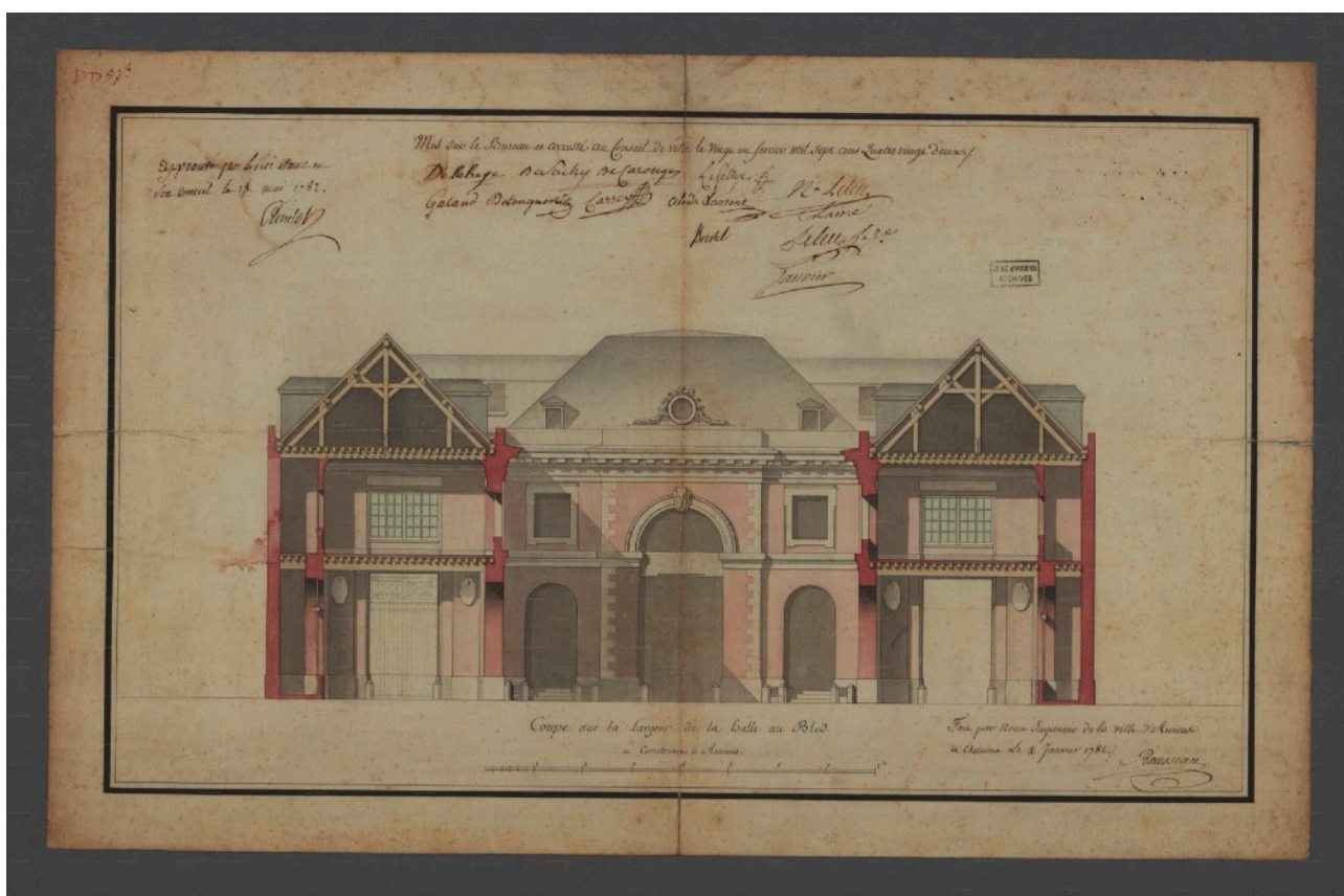
Archives municipales et communautaires d'Amiens, DD57_4, Jacques-Pierre-Jean ROUSSEAU, Coupe sur la longueur et coupe sur la largeur de la halle au bled à construire à Amiens , disponible en ligne sur la plateforme l'Armarium ( https://www.armarium-hautsdefrance.fr/document/19673 )
